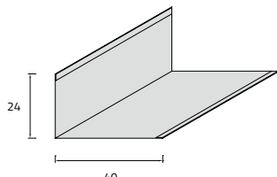
40 X 24 CP 50 aluminum 0.5/0.6 mm A 3002/B - A 3002/N - A 3002/M steel 0.5 mm
