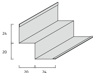
24 X 20 X 20 X 24 W 3003/B - W 3003/N - W 3003/M steel 0.5 mm
